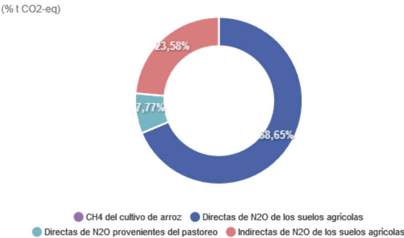
Fig. 6 Porcentaje según el tipo de emisiones GEI en agricultura (2019) Fuente: Huella de Carbono de los municipios andaluces. https://www.juntadeandalucia.es/medioambiente/portal/web/cambio-climatico/indice/-/asset_publisher/hdxWUGtQGkX8/content/huella-de-carbono-de-los-municipios-andaluces/20151 (24/07/2022)
