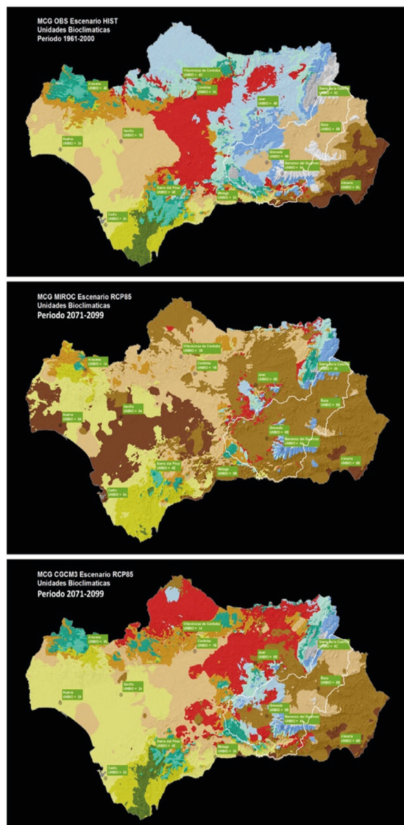
Ilustración 2. Clasificación bioclimática de Andalucía para los periodos: a) 1961-2000; b) 2071-2099 según MIROC en RCP85 (contexto más pesimista); c) 2071-2099 según CGCM3 en RCP85 (contexto más optimista).
