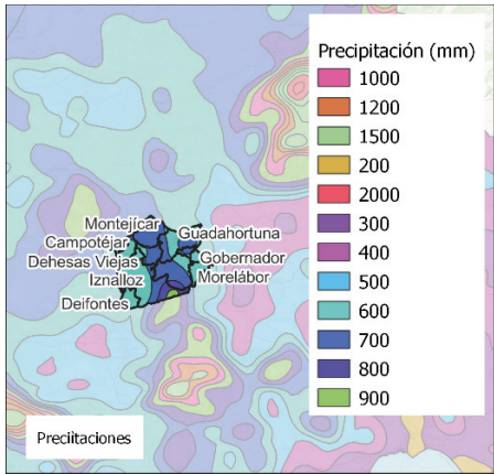
Ilustración 6: Precipitaciones anuales
