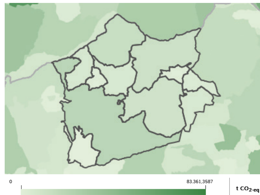
Fig. 8 Absorciones GEI
